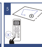
5 Кездейсоқ бағдар
